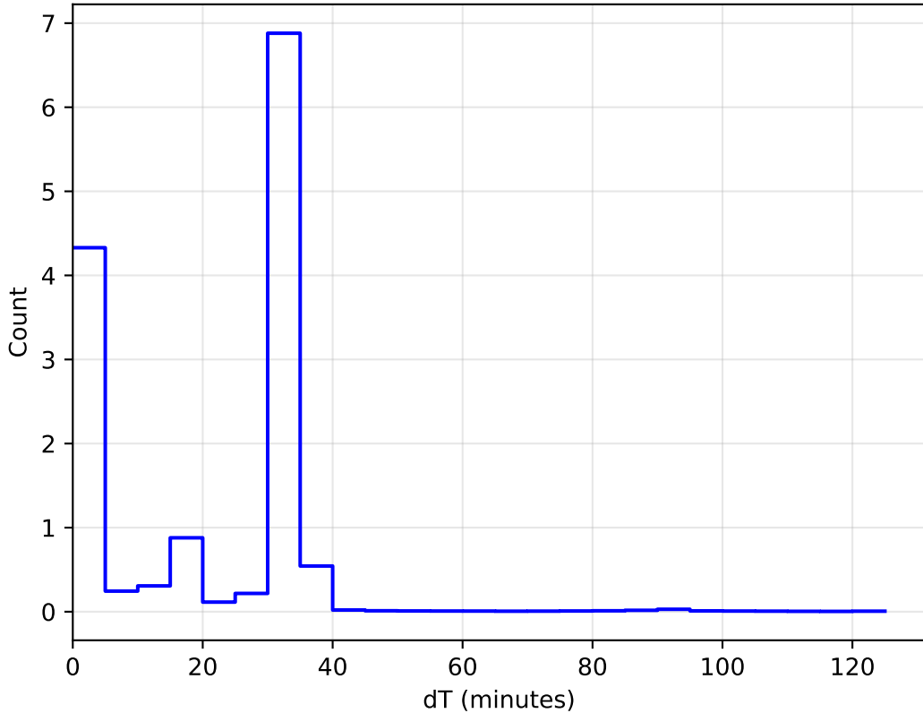
weather_cloudso10v3.4_10yrs All sky: DeltaT Histogram
