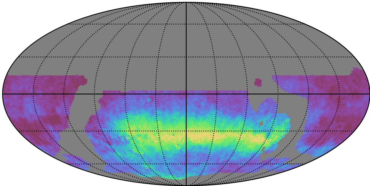
weather_cloudso10v3.4_10yrs WFD y band: AngleRms rotSkyPos
