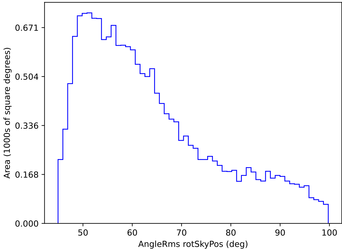
weather_cloudso10v3.4_10yrs WFD y band: AngleRms rotSkyPos
