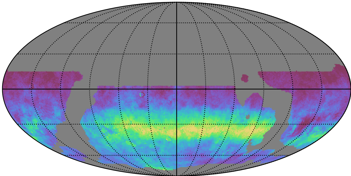
weather_cloudso10v3.4_10yrs WFD i band: AngleRms rotSkyPos
