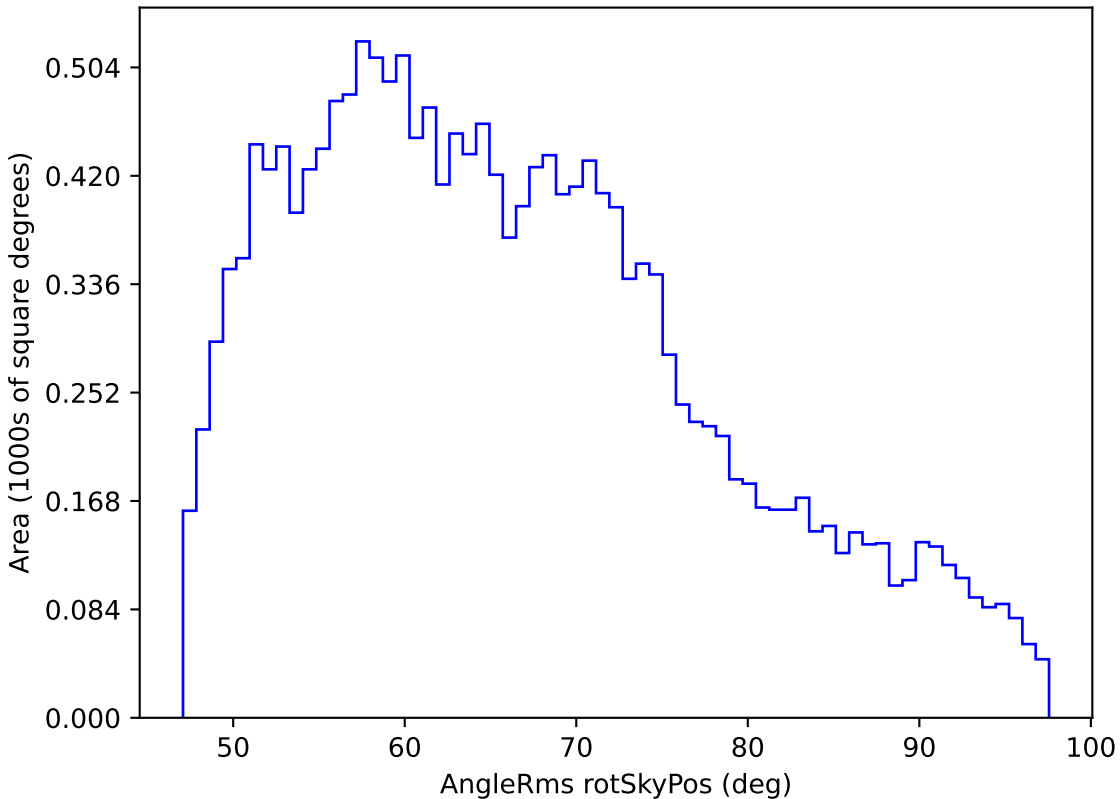
weather_cloudso10v3.4_10yrs WFD i band: AngleRms rotSkyPos
