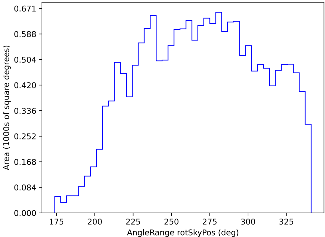
weather_cloudso10v3.4_10yrs WFD y band: AngleRange rotSkyPos
