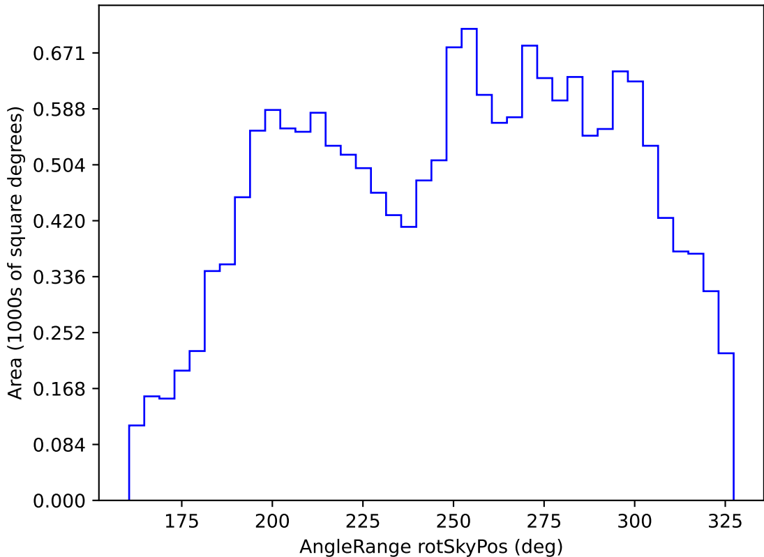
weather_cloudso10v3.4_10yrs WFD u band: AngleRange rotSkyPos
