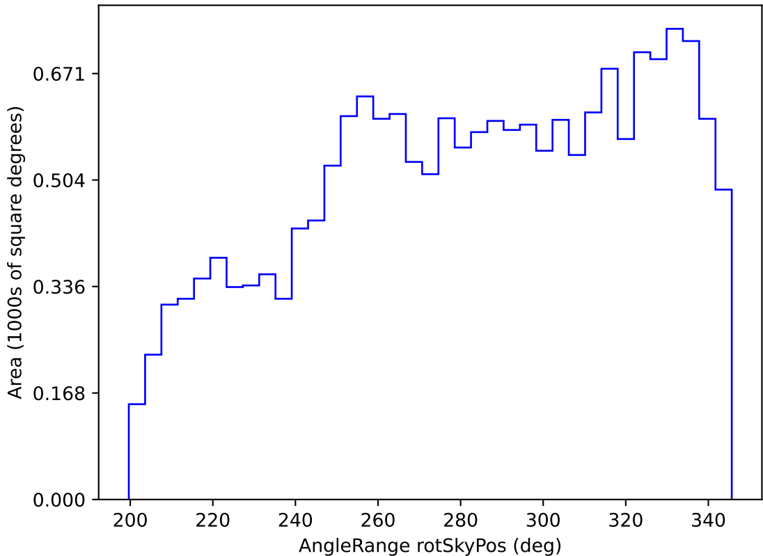
weather_cloudso10v3.4_10yrs WFD r band: AngleRange rotSkyPos
