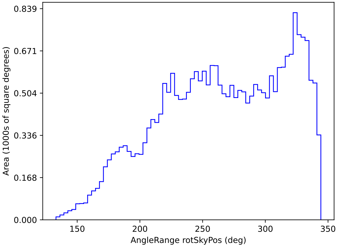
weather_cloudso10v3.4_10yrs All sky z band: AngleRange rotSkyPos
