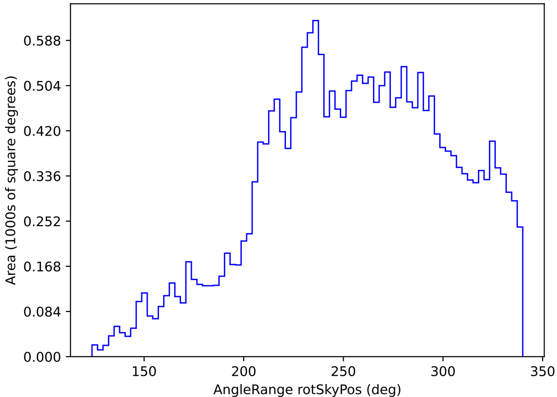
weather_cloudso10v3.4_10yrs All sky y band: AngleRange rotSkyPos
