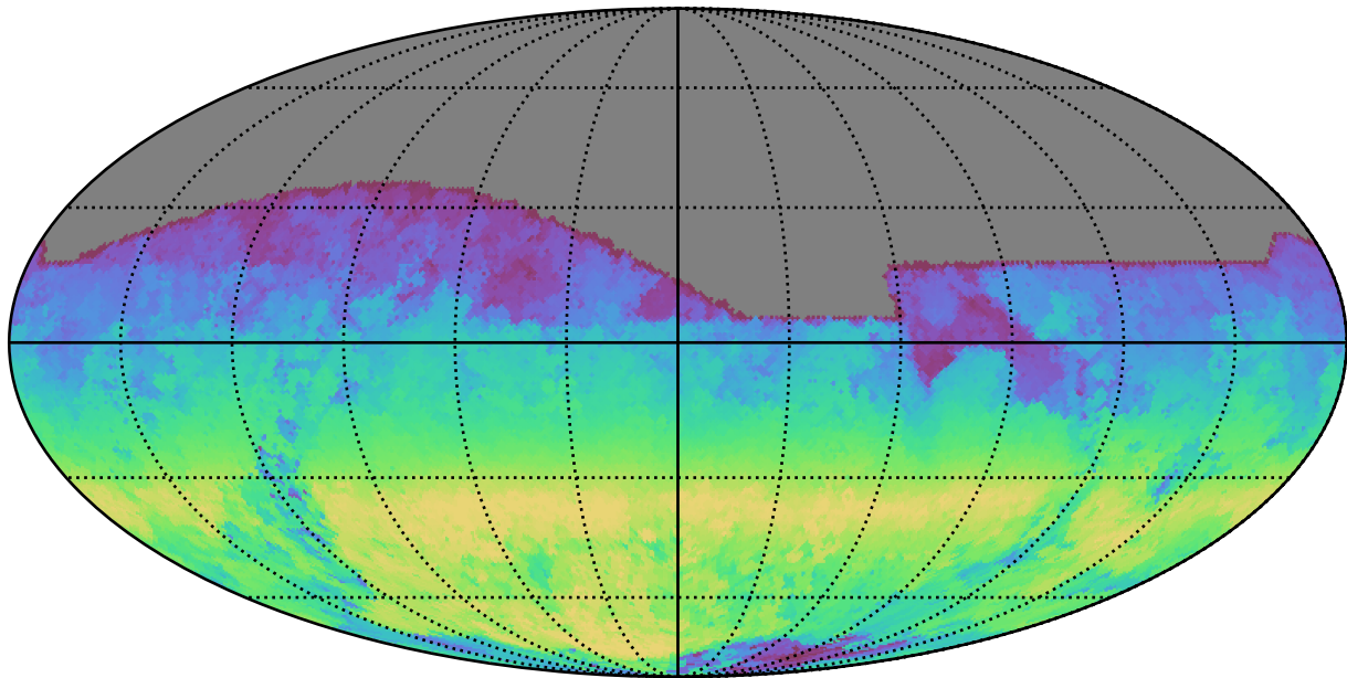
weather_cloudso10v3.4_10yrs All sky r band: AngleRange rotSkyPos
