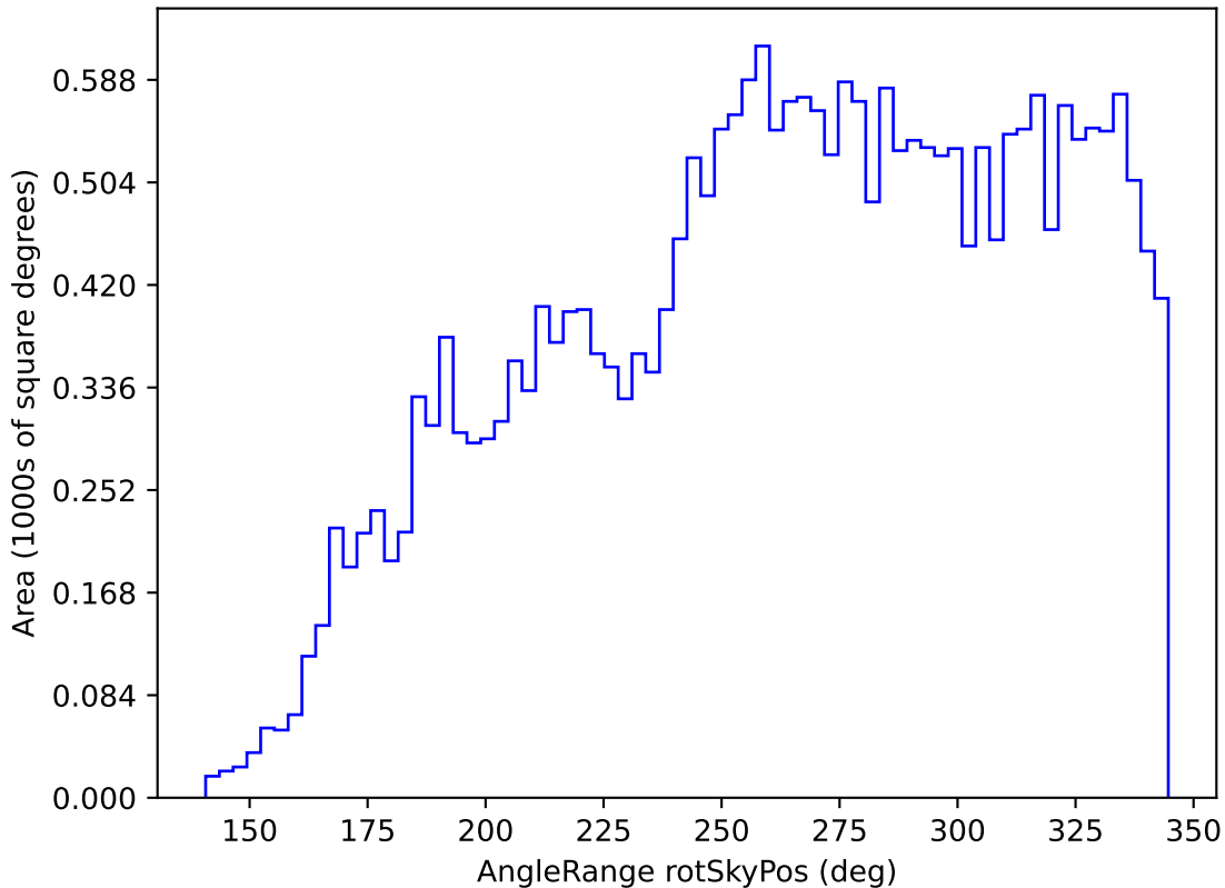
weather_cloudso10v3.4_10yrs All sky r band: AngleRange rotSkyPos
