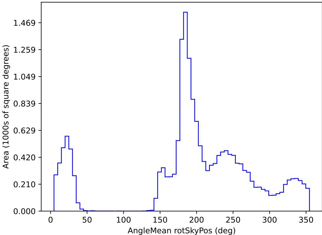
weather_cloudso10v3.4_10yrs WFD z band: AngleMean rotSkyPos
