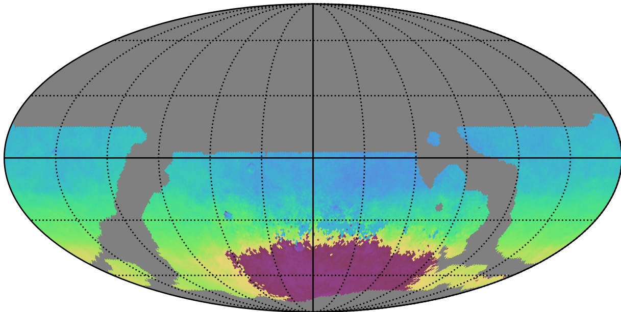
weather_cloudso10v3.4_10yrs WFD y band: AngleMean rotSkyPos
