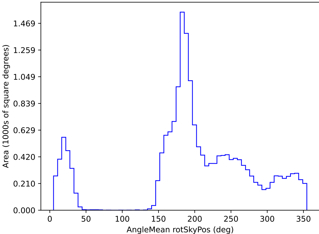
weather_cloudso10v3.4_10yrs WFD y band: AngleMean rotSkyPos
