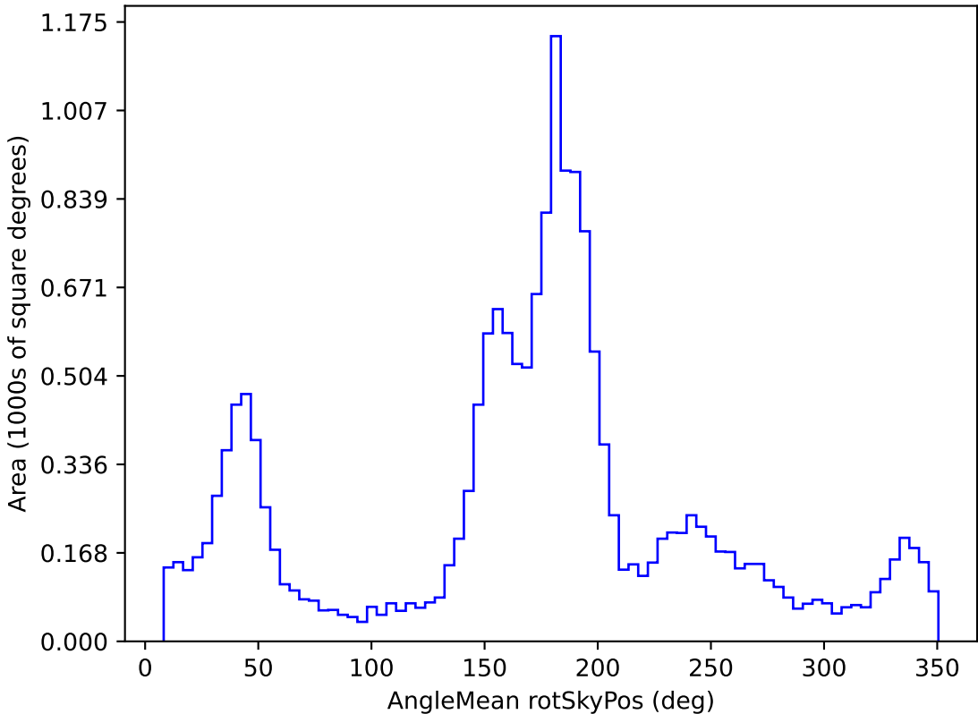
weather_cloudso10v3.4_10yrs WFD g band: AngleMean rotSkyPos
