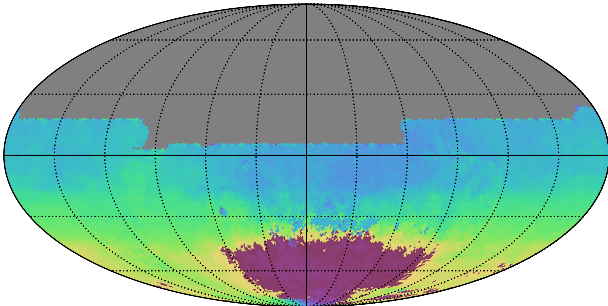
weather_cloudso10v3.4_10yrs All sky y band: AngleMean rotSkyPos
