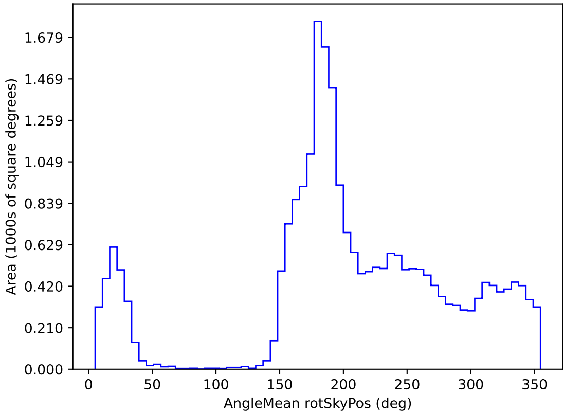
weather_cloudso10v3.4_10yrs All sky y band: AngleMean rotSkyPos
