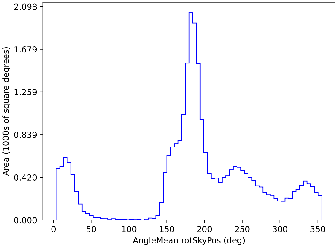
weather_cloudso10v3.4_10yrs All sky i band: AngleMean rotSkyPos
