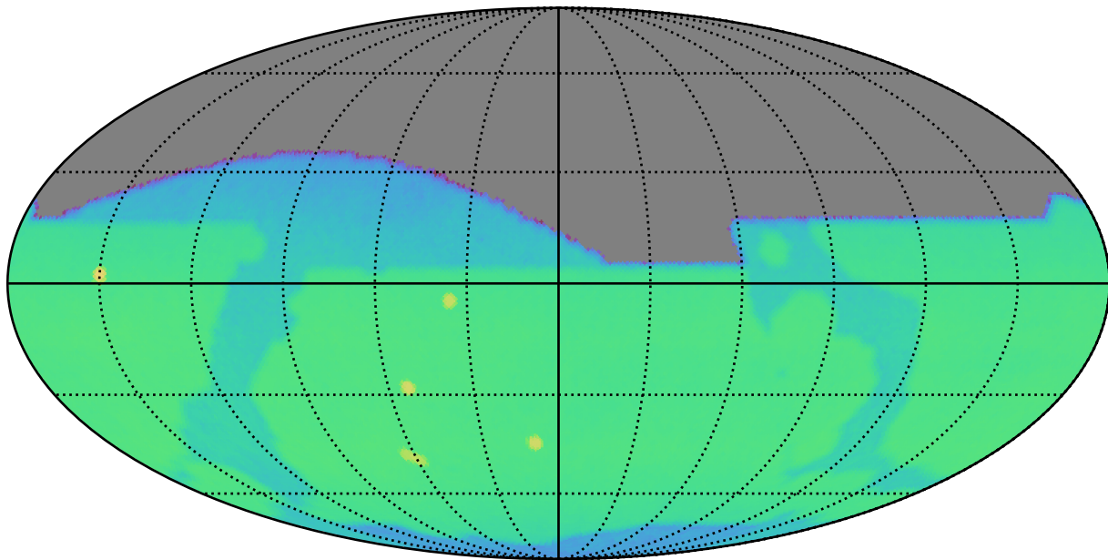
weather_cloudso10v3.4_10yrs i: CoaddM5
