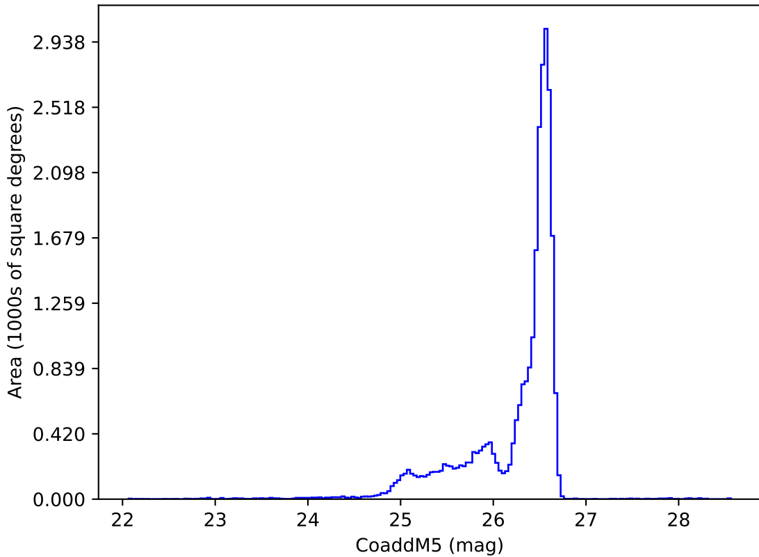
weather_cloudso10v3.4_10yrs i: CoaddM5
