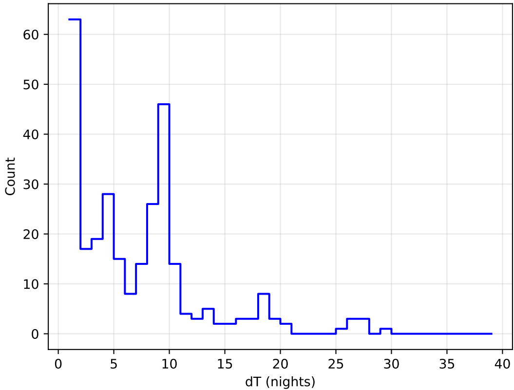
weather_cloudso10v3.4_10yrs all bands: DD:ELAISS1 Delta Nights Histogram
