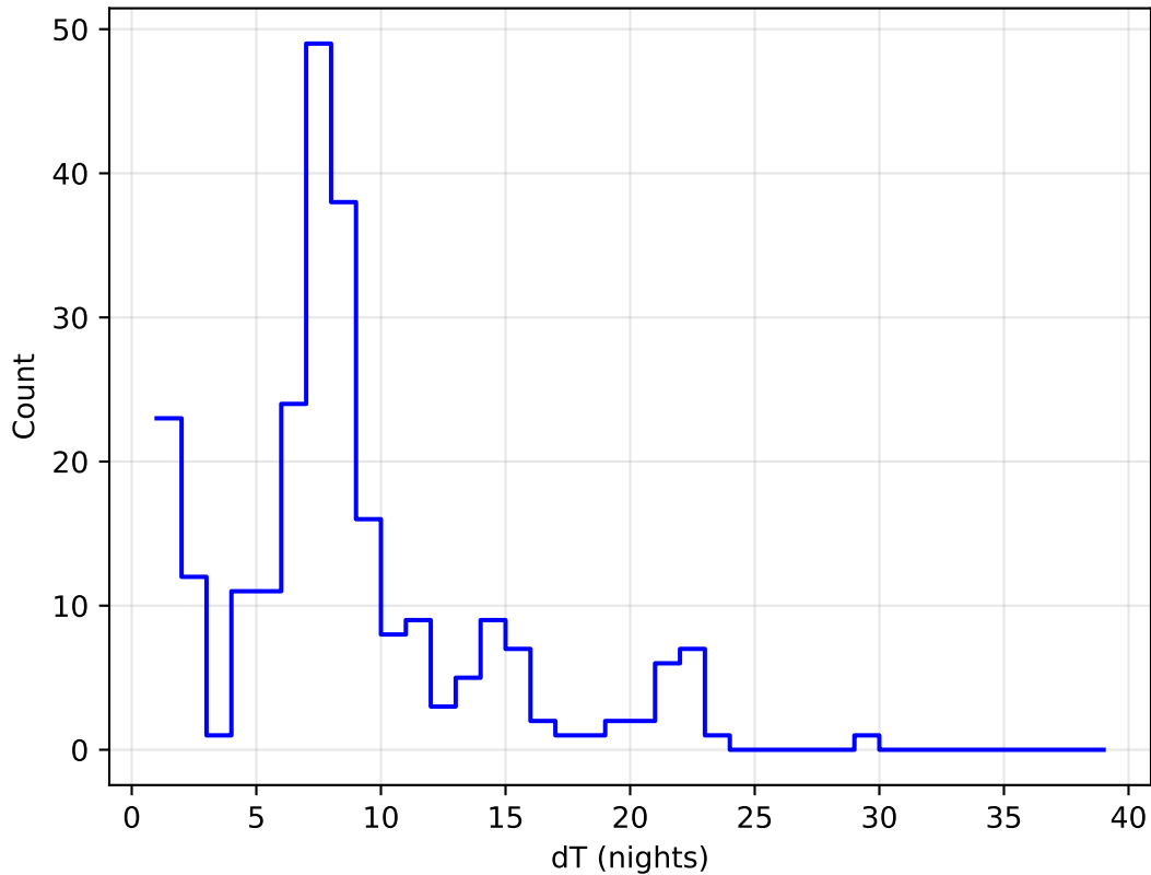
weather_cloudso10v3.4_10yrs all bands: DD:EDFS Delta Nights Histogram
