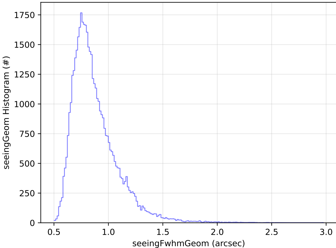
weather_cloudso0v3.5_10yrs Yr 1 y band: seeingGeom Histogram
