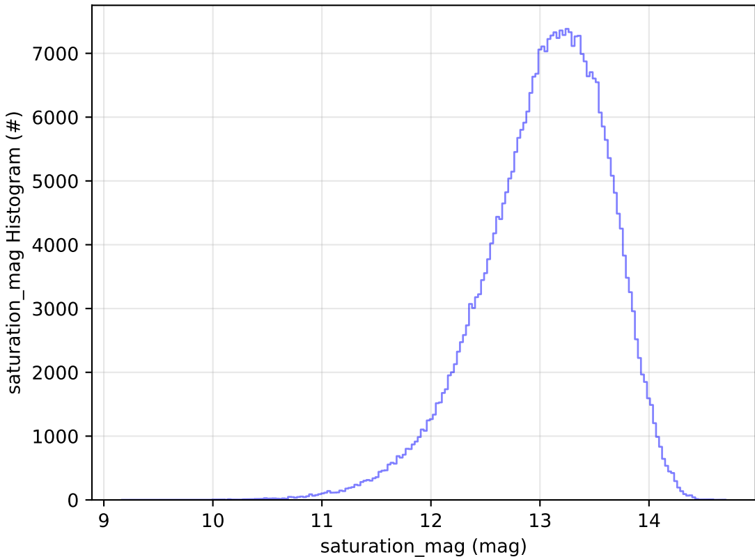
weather_cloudso0v3.5_10yrs WFD y band: saturation_mag Histogram
