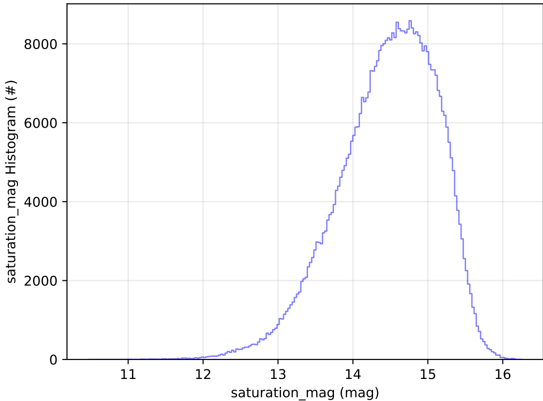
weather_cloudso0v3.5_10yrs WFD r band: saturation_mag Histogram
