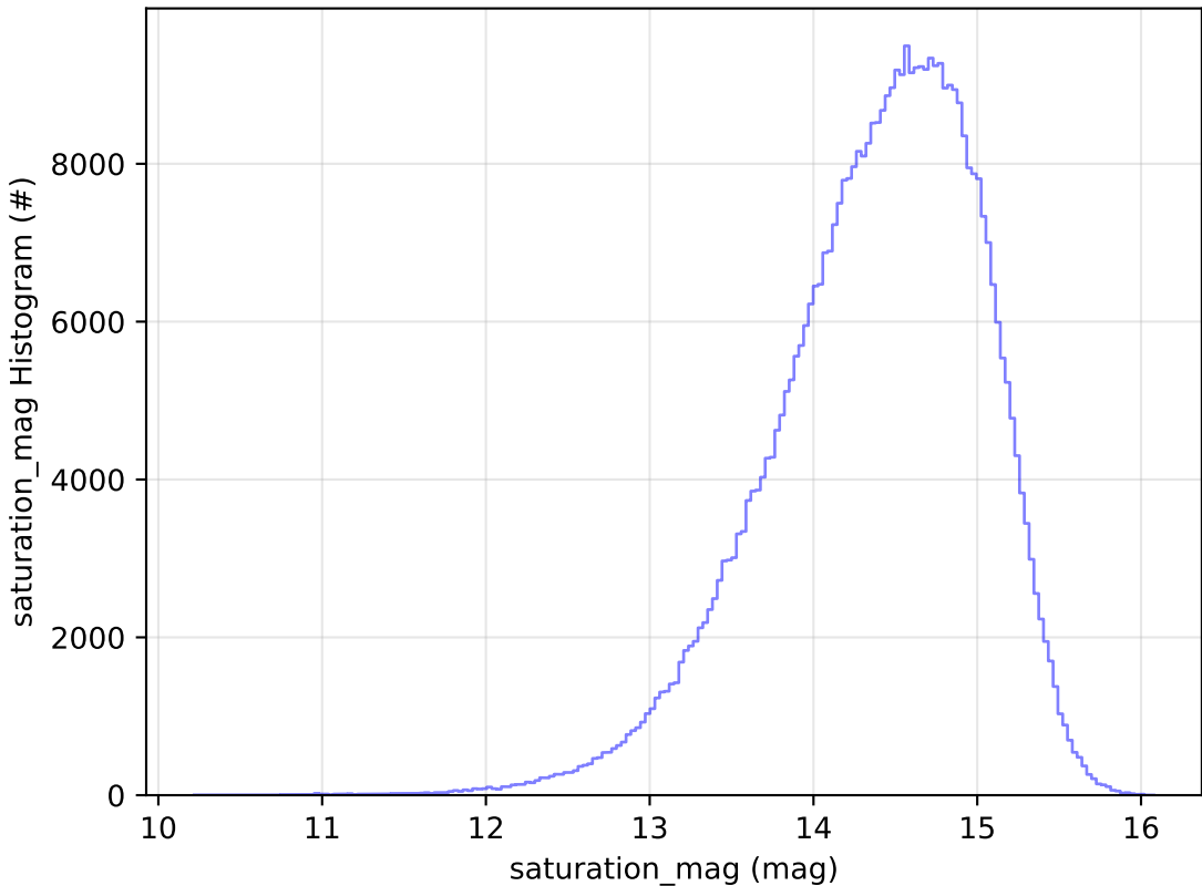
weather_cloudso0v3.5_10yrs WFD i band: saturation_mag Histogram
