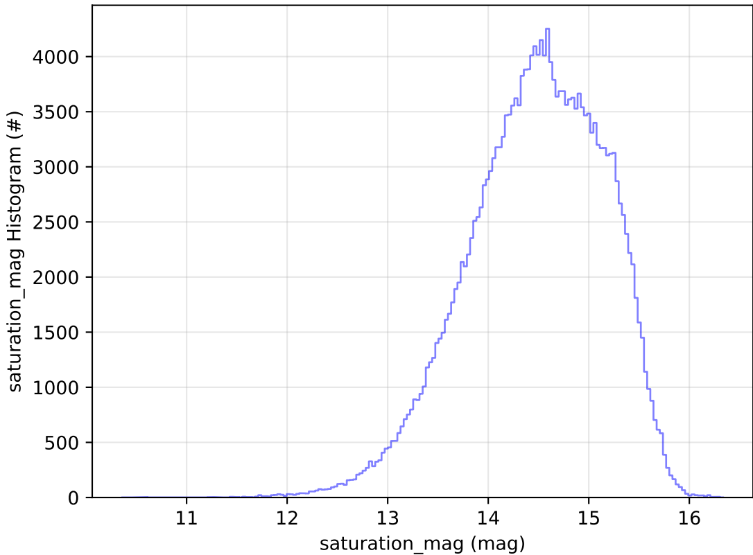
weather_cloudso0v3.5_10yrs WFD g band: saturation_mag Histogram
