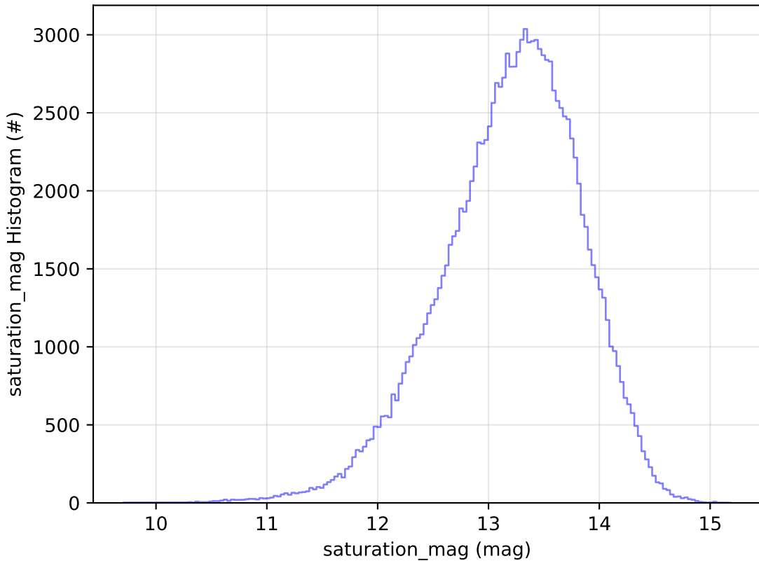
weather_cloudso0v3.5_10yrs All sky u band: saturation_mag Histogram
