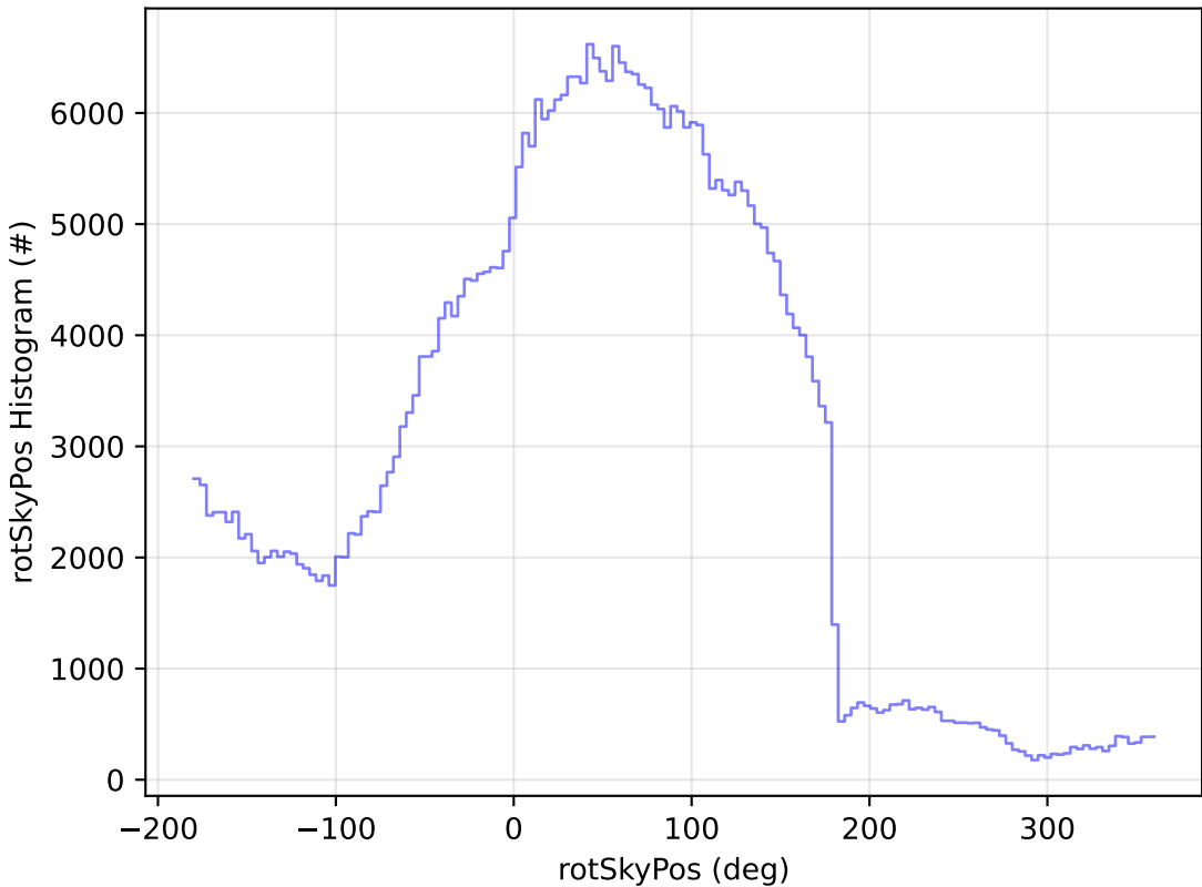
weather_cloudso0v3.5_10yrs WFD z band: rotSkyPos Histogram
