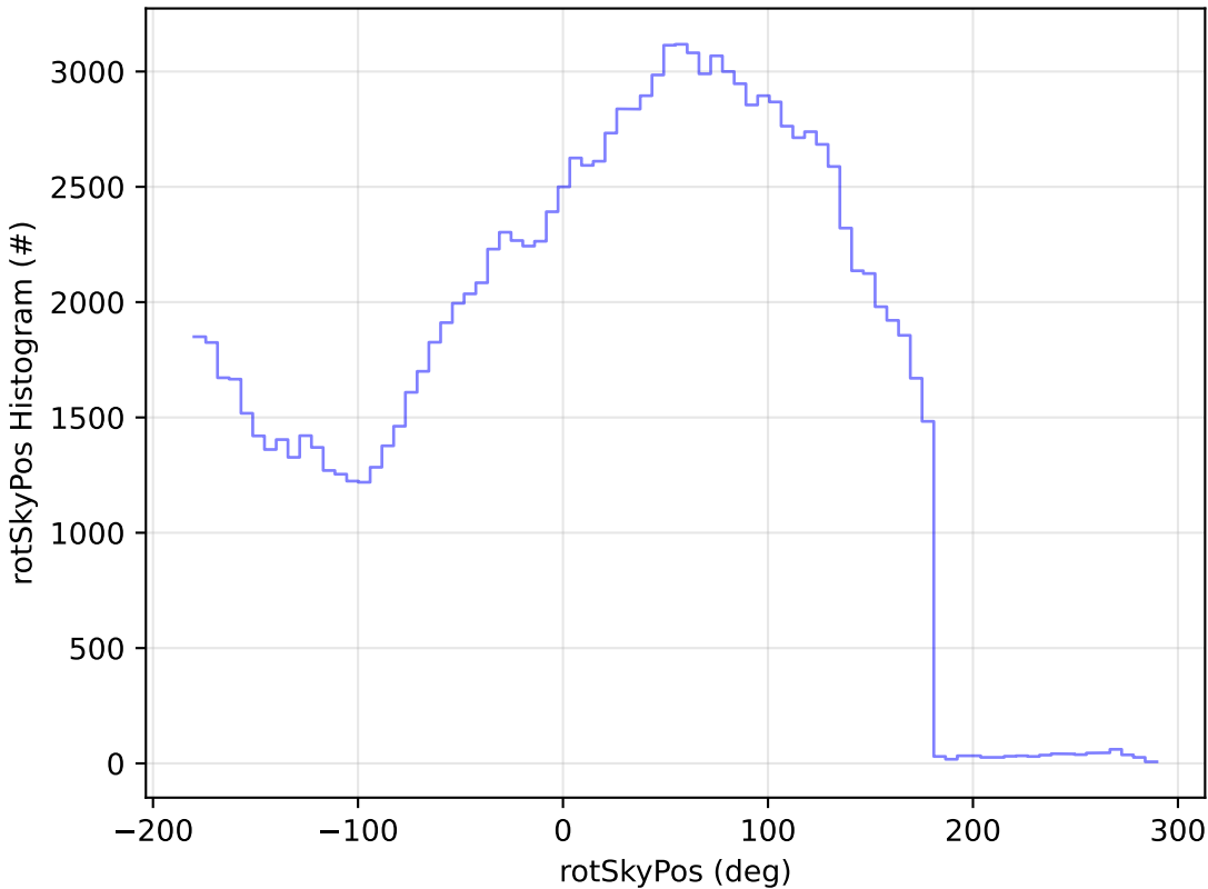
weather_cloudso0v3.5_10yrs WFD u band: rotSkyPos Histogram
