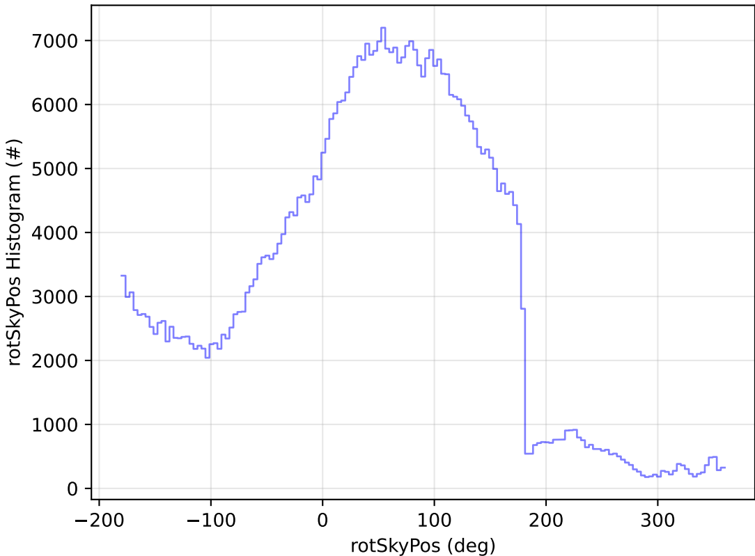
weather_cloudso0v3.5_10yrs WFD r band: rotSkyPos Histogram
