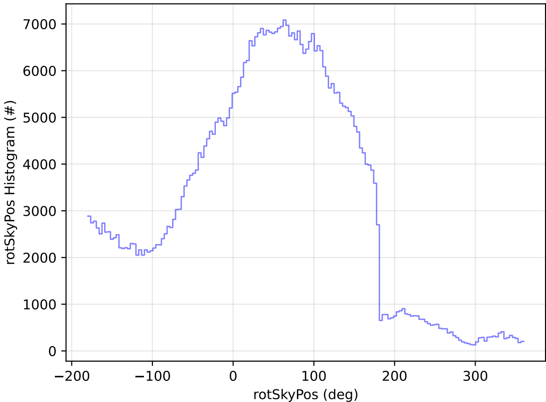
weather_cloudso0v3.5_10yrs WFD i band: rotSkyPos Histogram
