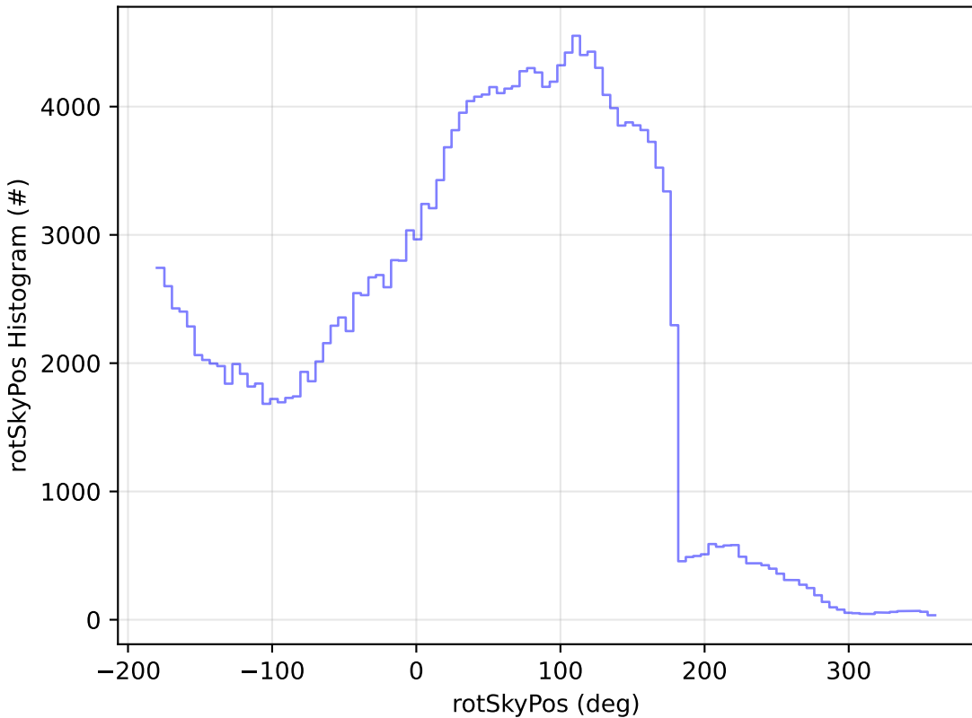
weather_cloudso0v3.5_10yrs WFD g band: rotSkyPos Histogram
