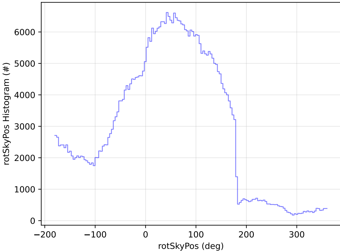
weather_cloudso0v3.5_10yrs All sky z band: rotSkyPos Histogram
