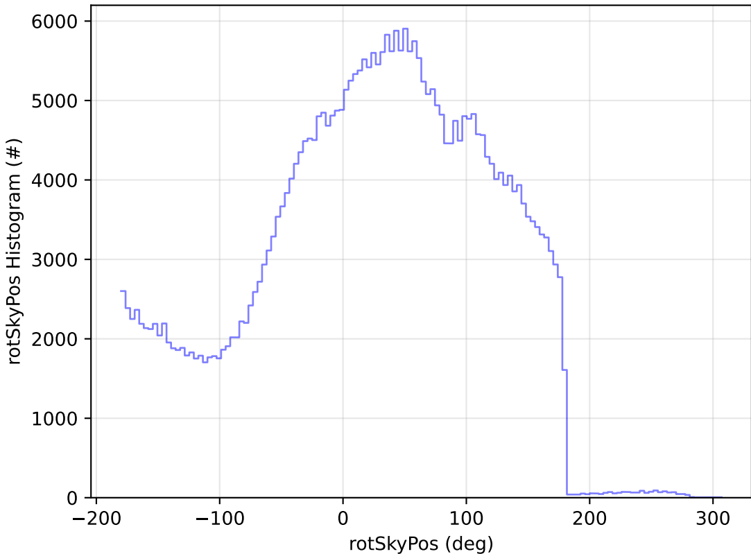
weather_cloudso0v3.5_10yrs All sky y band: rotSkyPos Histogram
