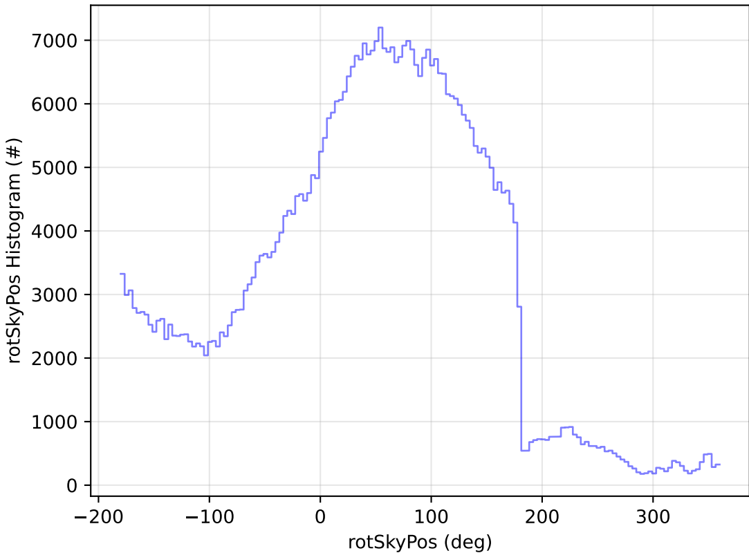
weather_cloudso0v3.5_10yrs All sky r band: rotSkyPos Histogram
