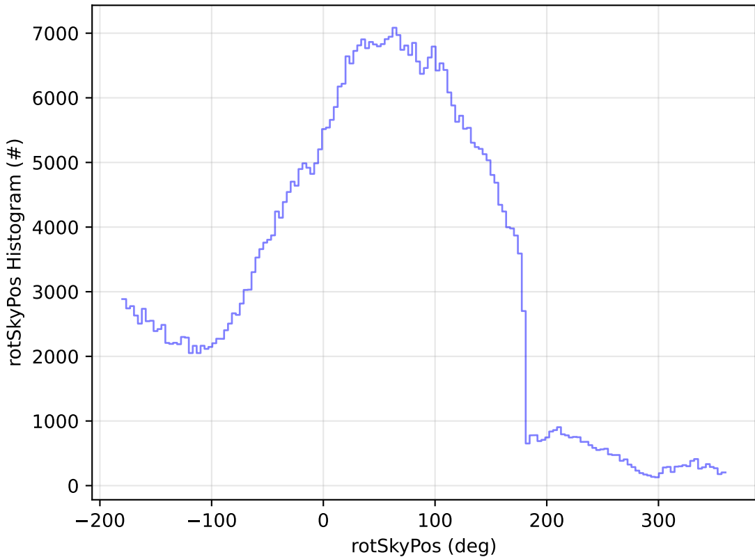
weather_cloudso0v3.5_10yrs All sky i band: rotSkyPos Histogram
