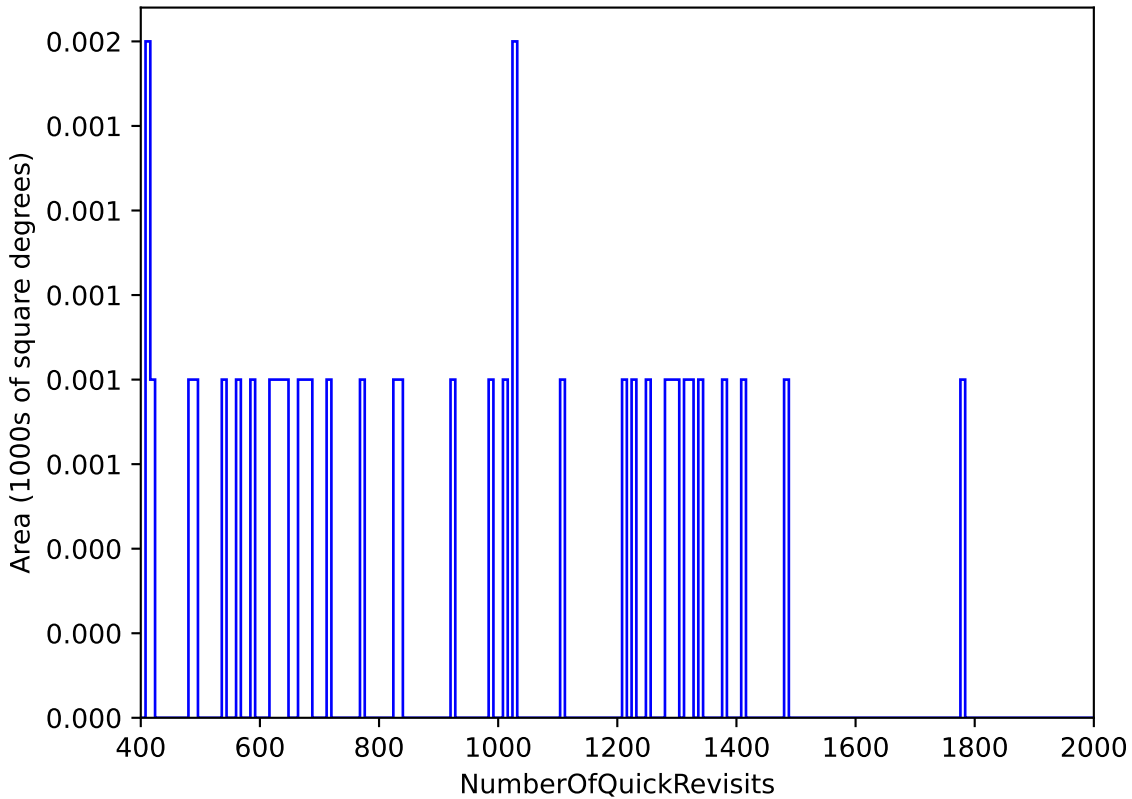
weather_cloudso0v3.5_10yrs WFD: NumberOfQuickRevisits
