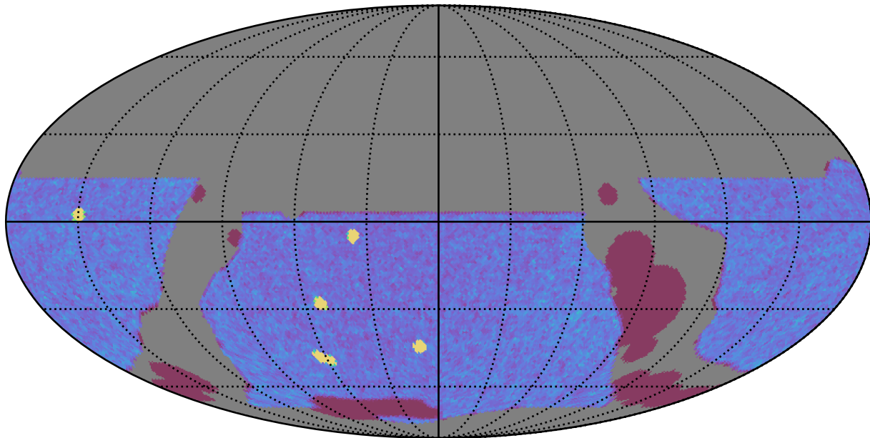
weather_cloudso0v3.5_10yrs WFD y band: NVisits
