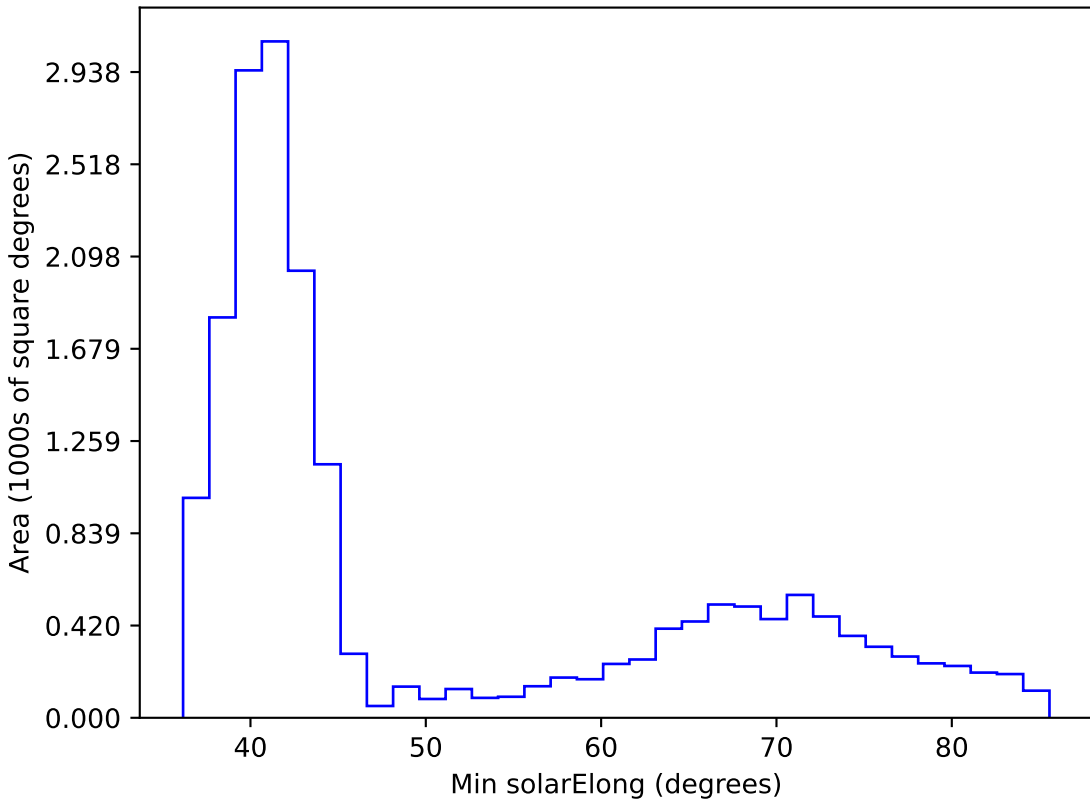
weather_cloudso0v3.5_10yrs WFD i band: Min solarElong
