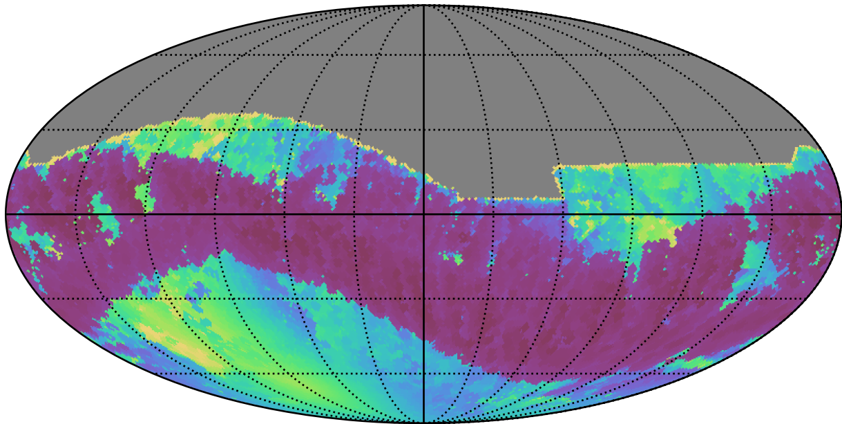
weather_cloudso0v3.5_10yrs All sky i band: Min solarElong
