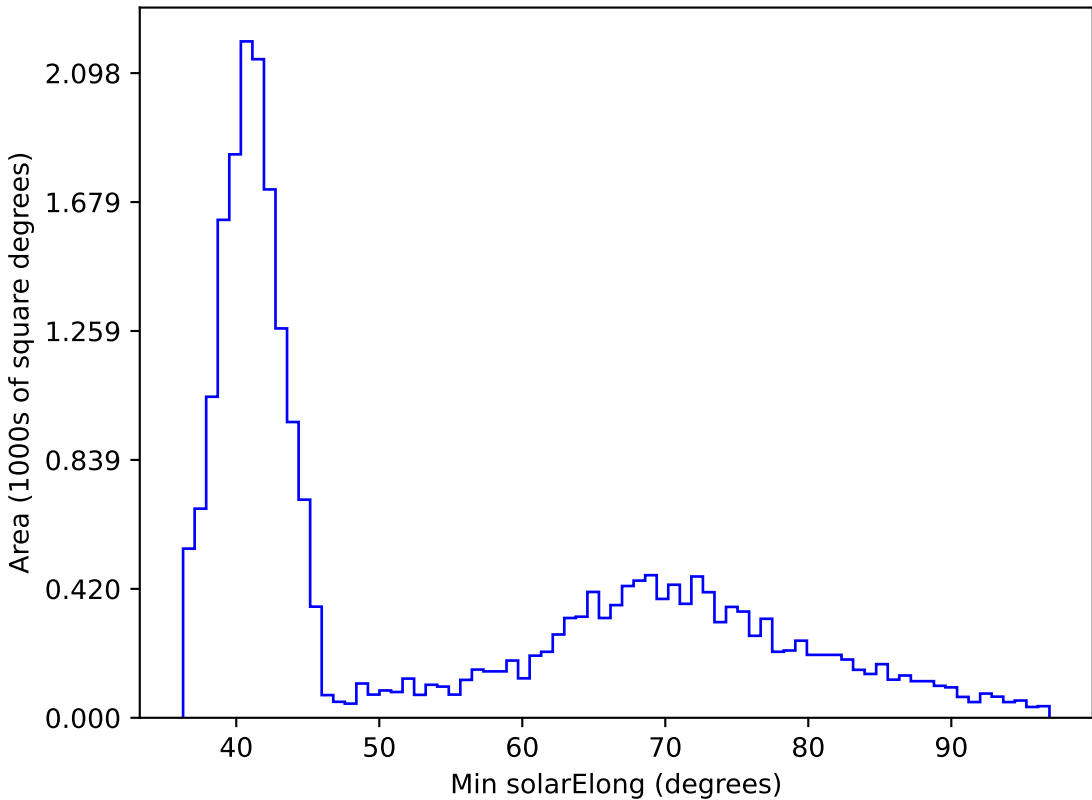
weather_cloudso0v3.5_10yrs All sky i band: Min solarElong
