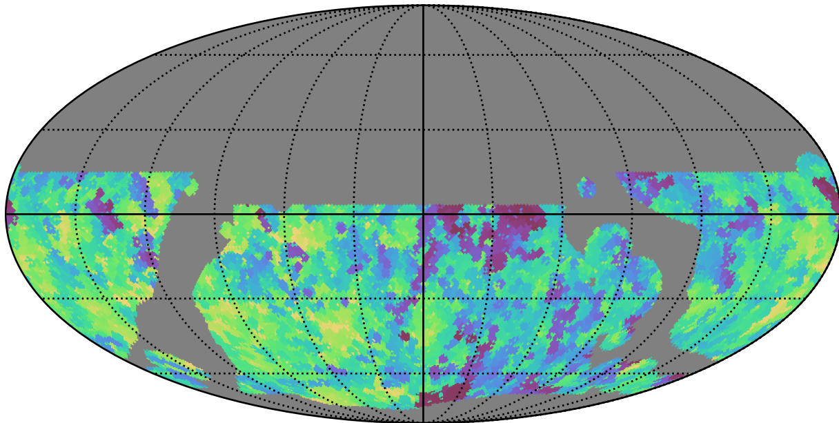
weather_cloudso0v3.5_10yrs WFD z band: Min saturation_mag
