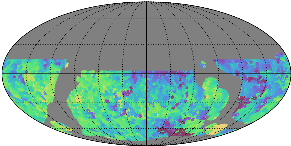
weather_cloudso0v3.5_10yrs WFD y band: Min saturation_mag
