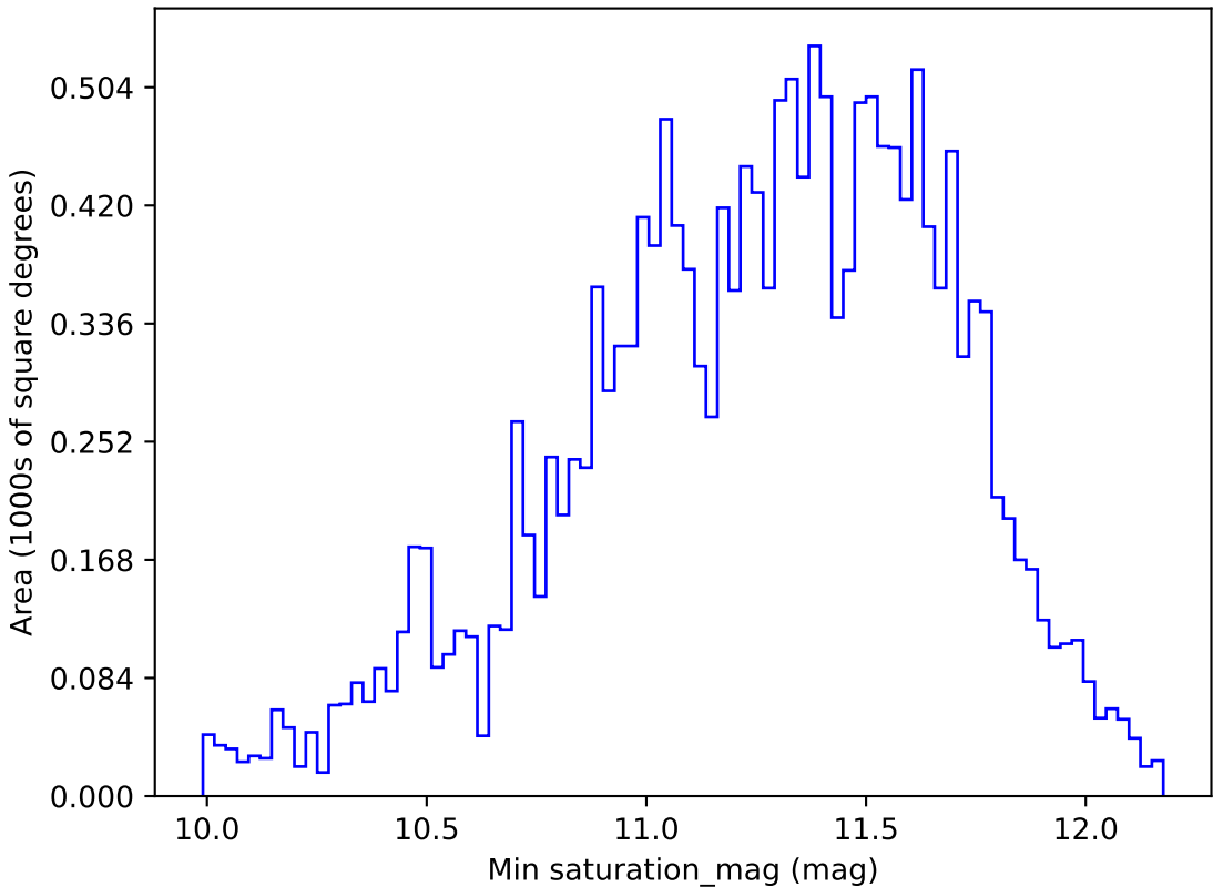
weather_cloudso0v3.5_10yrs WFD y band: Min saturation_mag
