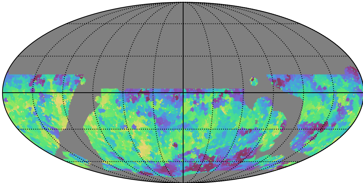
weather_cloudso0v3.5_10yrs WFD u band: Min saturation_mag
