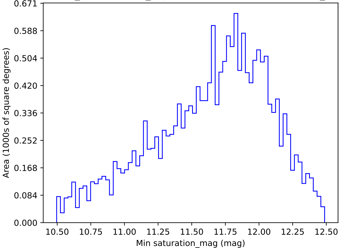
weather_cloudso0v3.5_10yrs WFD u band: Min saturation_mag
