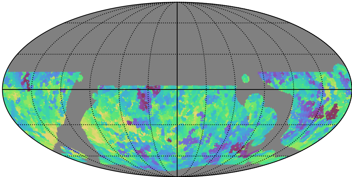
weather_cloudso0v3.5_10yrs WFD r band: Min saturation_mag
