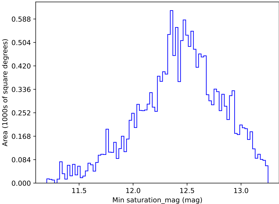
weather_cloudso0v3.5_10yrs WFD r band: Min saturation_mag
